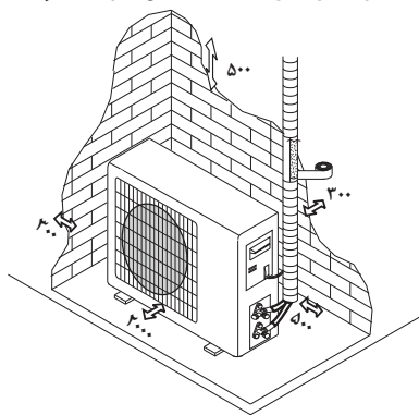
حداقل فضایی (میلی‌متر) که باید مطابق شکل لحاظ شود.
