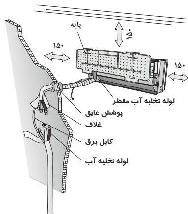
حداقل فضایی (میلی‌متر) که باید مطابق شکل لحاظ شود.
