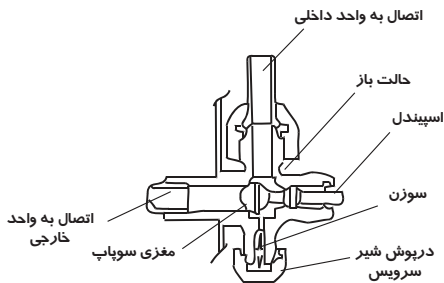
نمودار شیر سه‌طرفه
